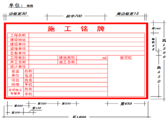
图 10 建筑工地施工铭牌
